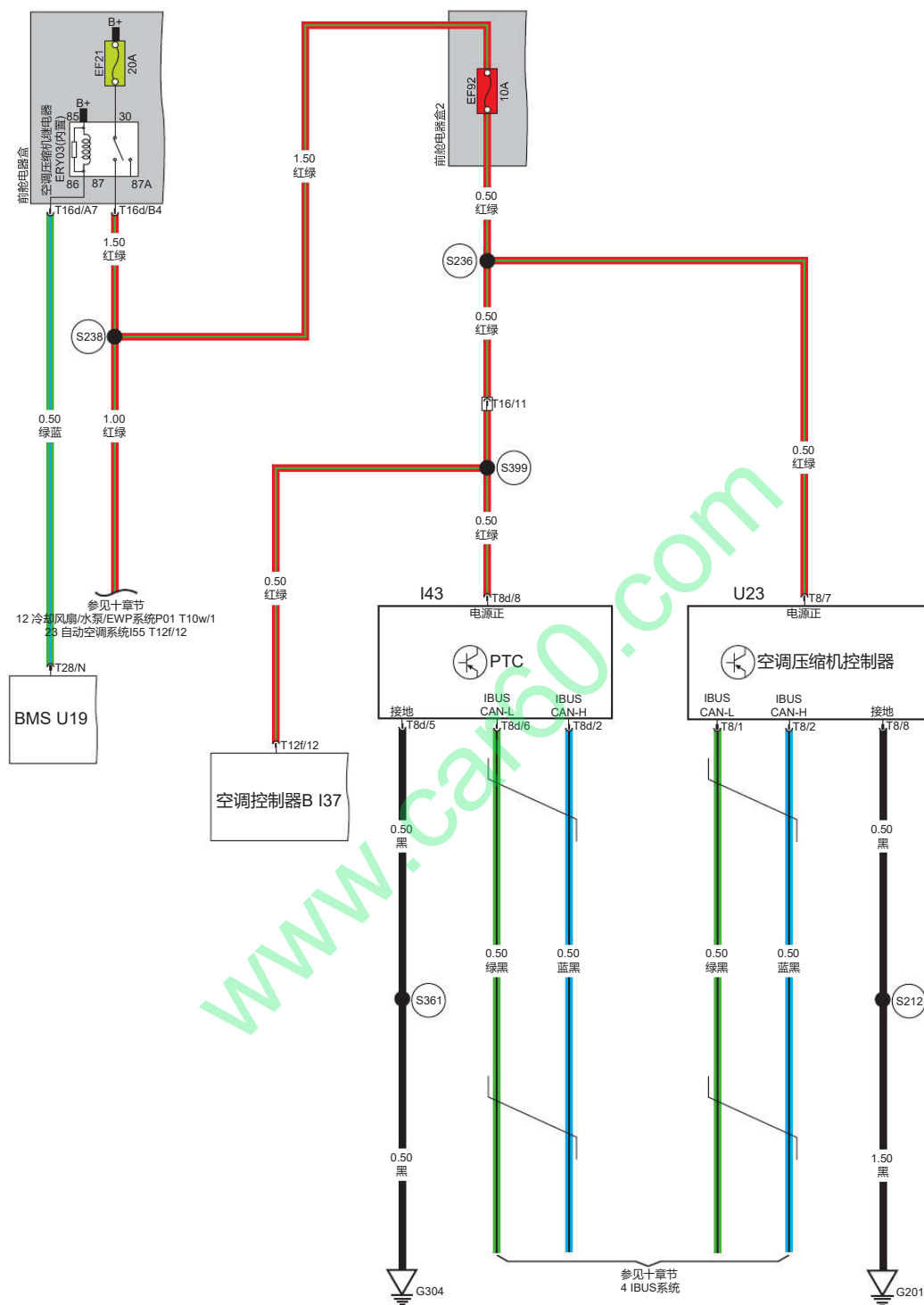
PTC 电加热控制 /EAS 电动压缩机控制系统接线图 C40D-DL-1016
